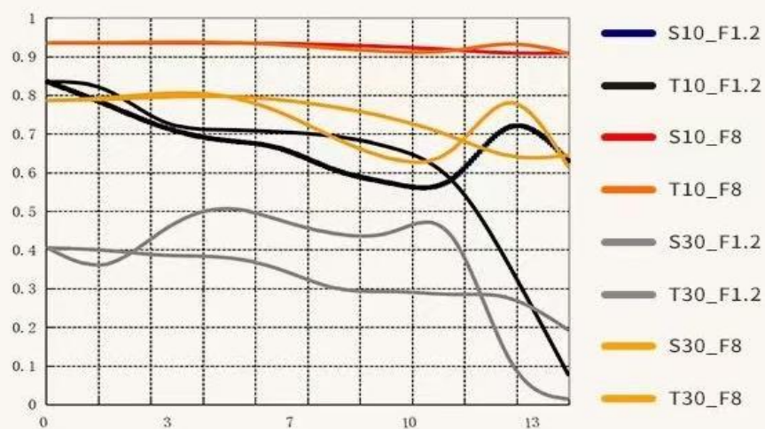
• MTF参数图
